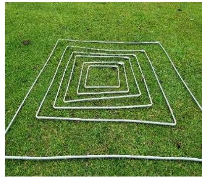
شکل ۲: نحوه استقرار پلات‌های هم‌مرکز نمونه‌برداری با ابعاد مختلف (۰/۵، ۱، ۲، ۳، ۵ و ۱۰ متر مربع)
